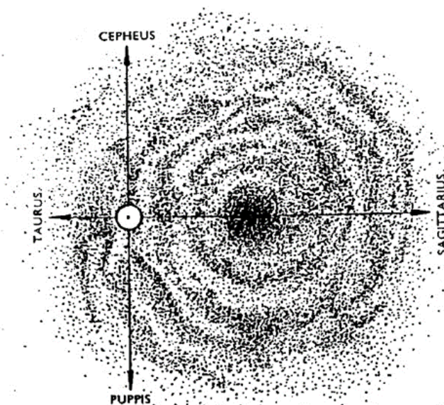
Galaxisunk (a Tejútrendszer) vázlatos képe
