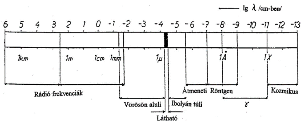
Elektromágneses hullámok spektruma.
