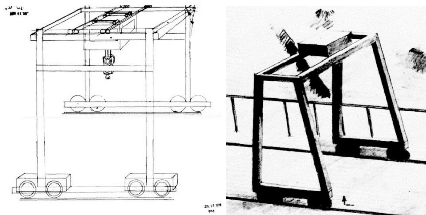
Balra: Pat Price pszichikus benyomásainak a rajza egy daru állványzatról a titkos szovjet R&D telepen Szemipalatyinszknál, 16,000 km-es távolságból. Jobbra: A tényleges nyolckerekű daru.
